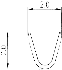
A-A SECTION
